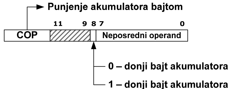
Слика 3.3 Непосредно адресирање
